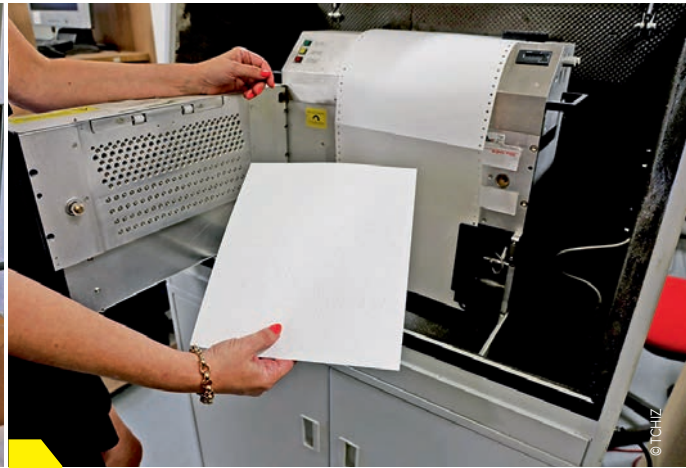
L'impression des textes est réalisée en recto verso par une embosseuse.
